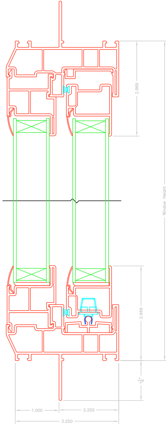
Section A-A
